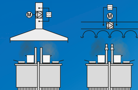
Gasgerät Typ B / Gas appliance type B
