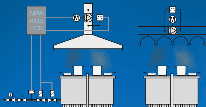
Gasgerät Typ A / Gas appliance type A
