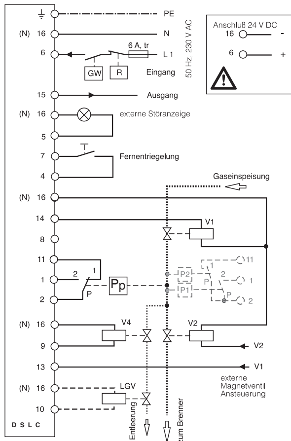
Anschlußplan DSLC für direkte Ventilkontrolle V1 mit Hilfsventil V4 oder LGV (zu Prinzipschema 3)
