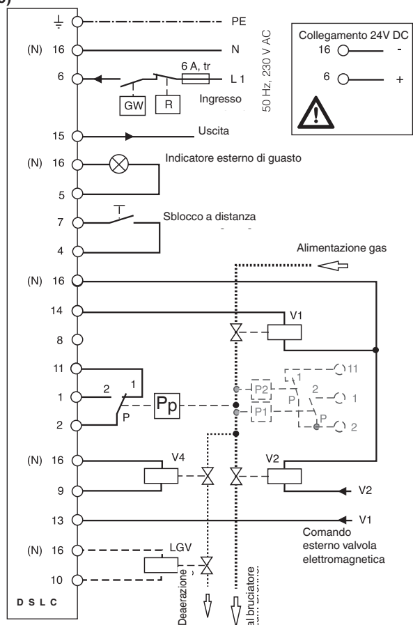
Schema dei collegamenti DSLC per controllo diretto valvola V1 con valvola ausiliaria V4 o LGV (v. Schema di funzionamento 3)
