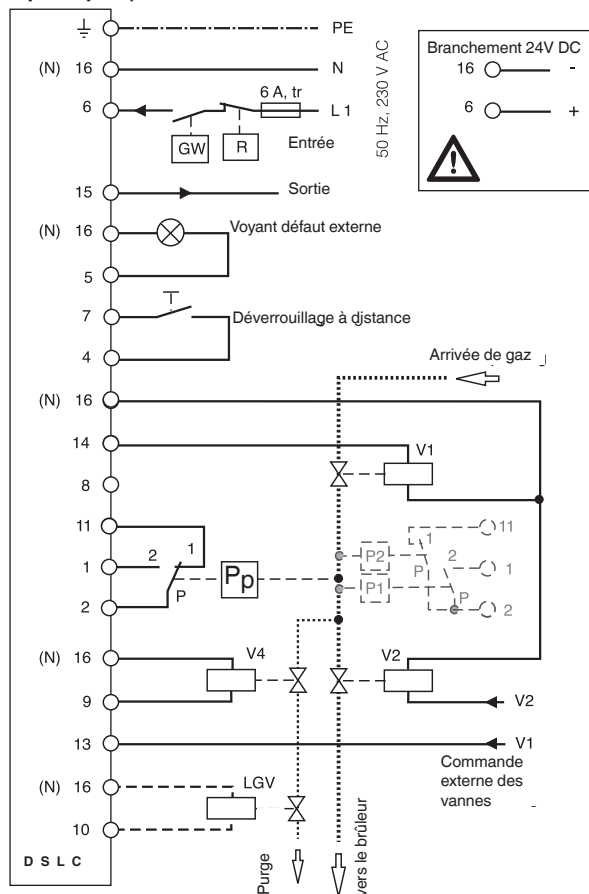
Schéma de branchement DSLC pour le contrôle direct de vanne V1 avec vanne auxiliaire V4 ou LGV (va avec le schéma de principe 3)
