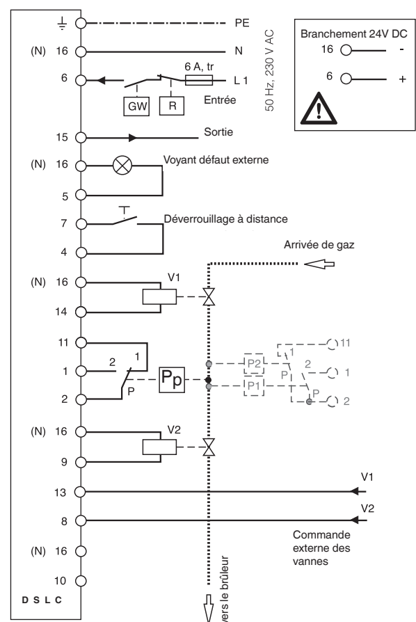
Schéma de branchement DSLC pour le contrôle direct de vanne V1, V2 (va avec le schéma de principe 4)
