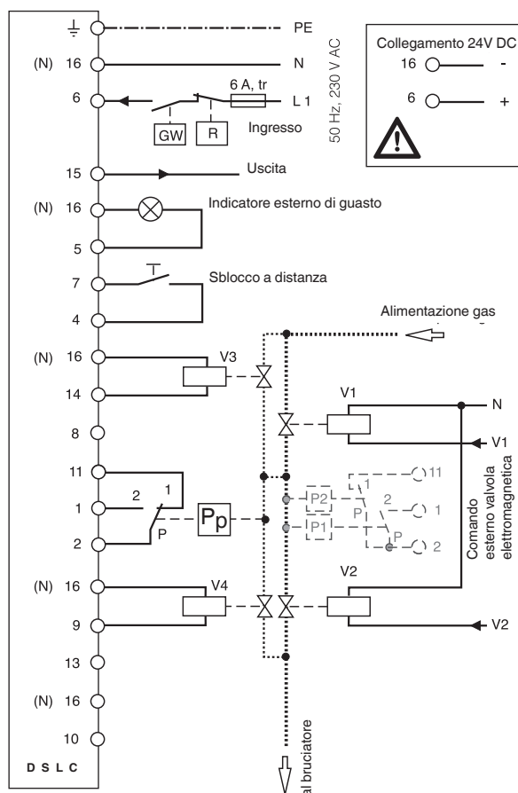
Schema dei collegamenti DSLC per controllo diretto valvole V1, V2 (v. Schema di funzionamento 4)
